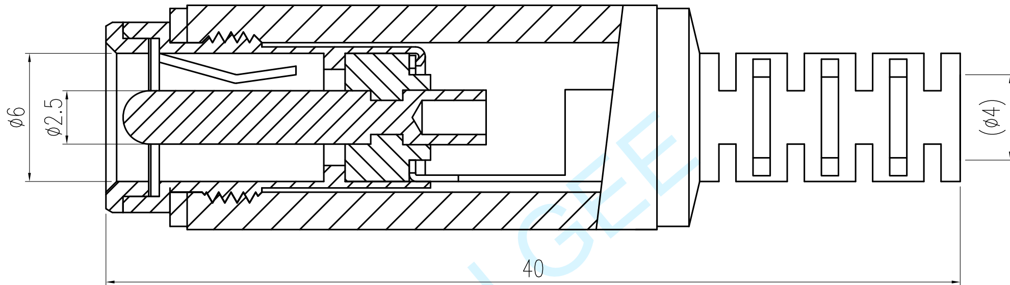
JA5525A
