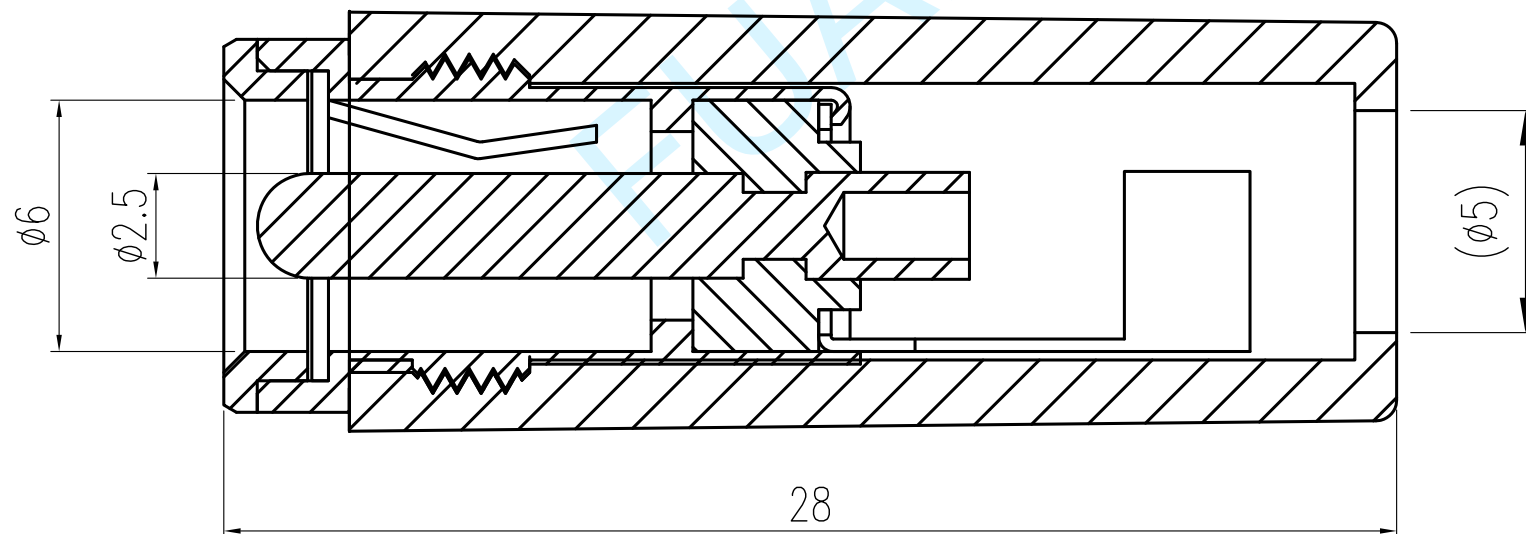
JA5525A-1
